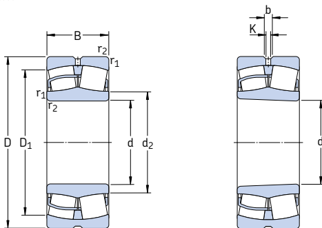
Alésage cylindrique
