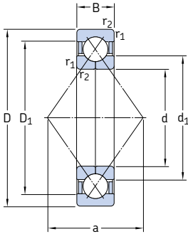
Exécution de base
