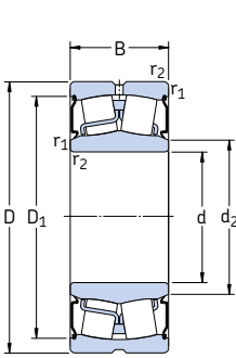
Alésage cylindrique
