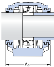
Joint à chicane Exécution S
