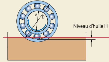
Niveau d'huile dans un bain d'huile
