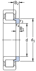
Bague d'épaulement
