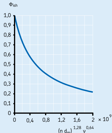
Facteur modérateur "cisaillement-échauffement" du lubrifiant
