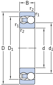
Alésage cylindrique
