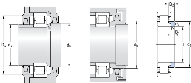
Bague d'épaulement
