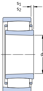
Alésage conique
