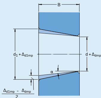
Diamètre maximal théorique d_1 = d + \frac{1}{30} \times B
