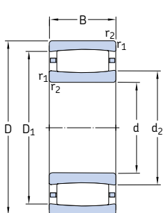
Alésage cylindrique
