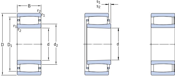
Alésage cylindrique
