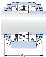
Joints à chicane Exécution S
