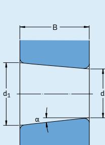
Demi-angle de cône 1:30 \alpha = 0^\circ 57' 17,4''
