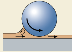
Flux de retour du lubrifiant
